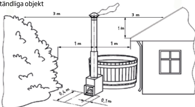
Minsta säkerhetsavstånd mellan vedeldade badtunnor och lättantändliga objekt
